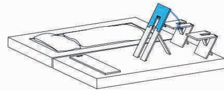
TISCHPLATTE INCL. TISCHBEINE RUNTERKLAPPEN IN FÜHRUNGSNUT
