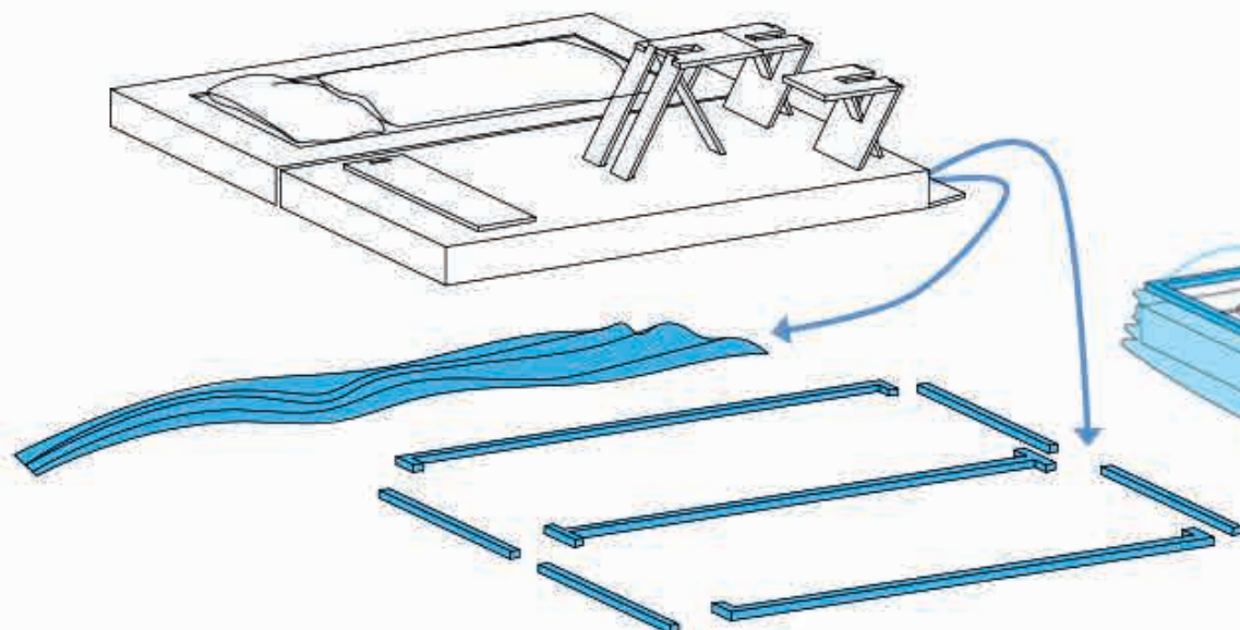
VORHANGTEILE AUS SEITENFACH NEHMEN UND ZUSAMMENBAUEN
